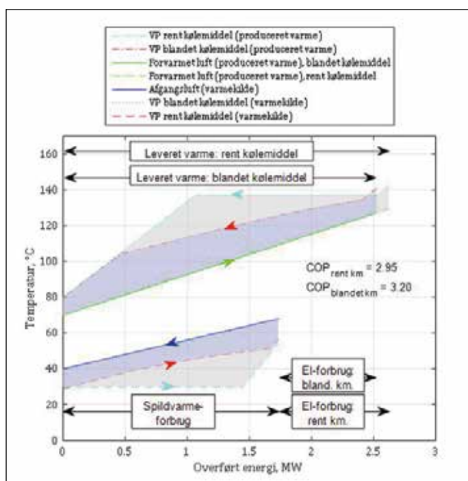
Figur 4. Enthalpi-Temperaturdiagram for rent og blandet kølemediel i varmepumpe for udnyttelse af overskudsvarme i mælkepulverproduktion (VP: varmepumpe).
